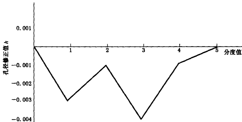
图 B.1 孔径修正值与分度值关系
