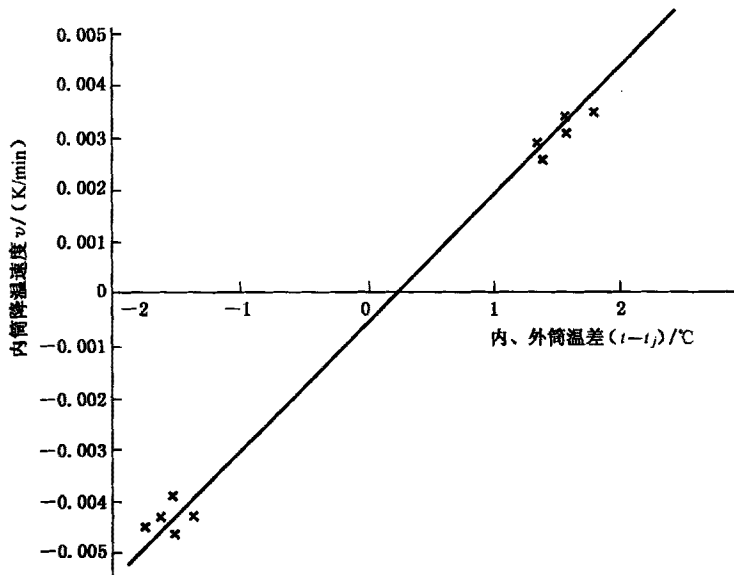
图 1 v \sim (t-t_j) 关系曲线
